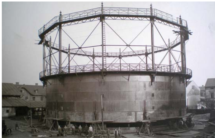
Montáž plynojemu v roce 1910.
